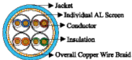
Cat6A S/FTP
